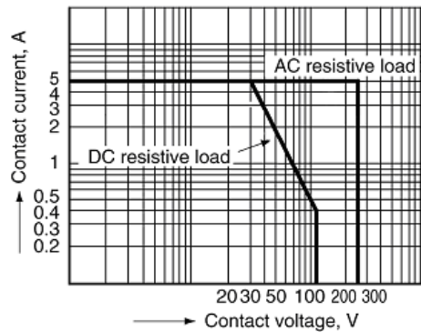
Maximale Schaltleistung
