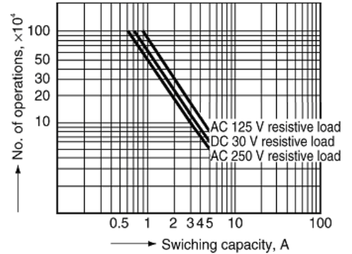
Lebensdauer
